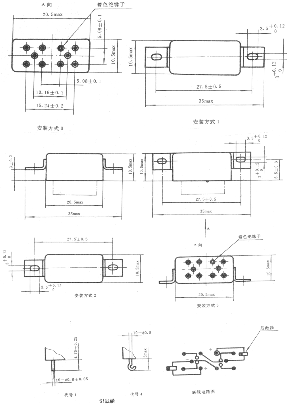
图 1 外形、安装、引出端及底视电路图
